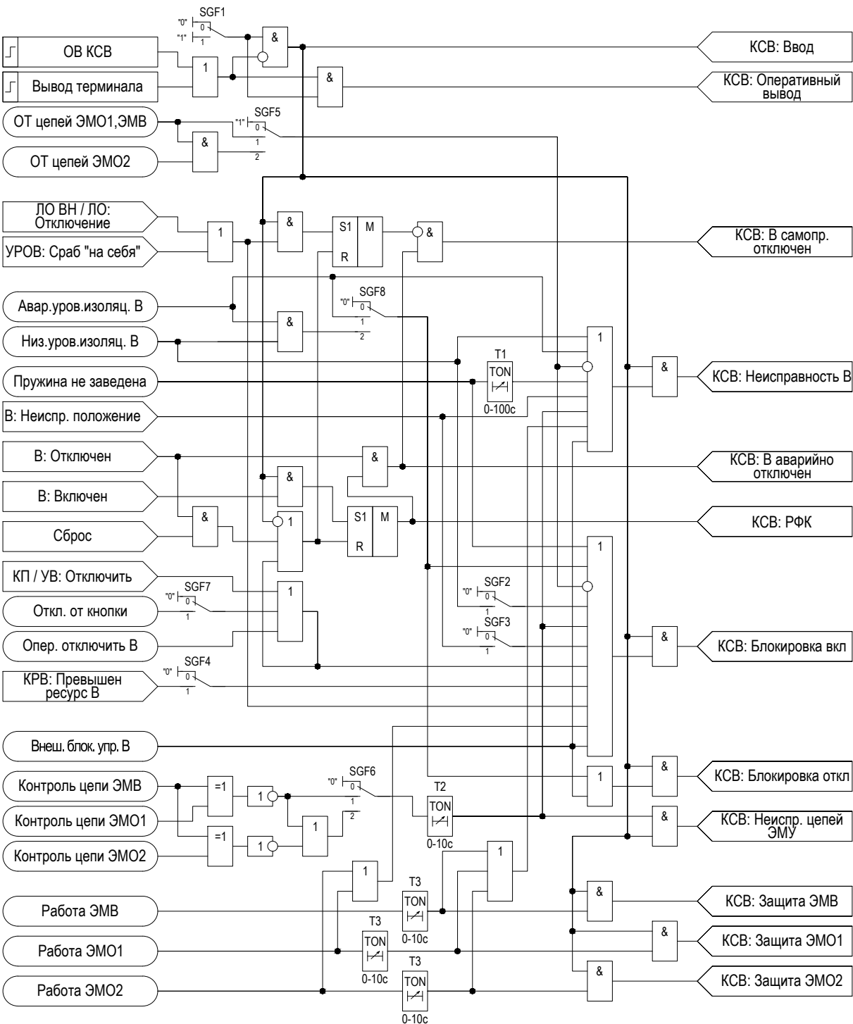
Рисунок 2.30 – Функциональная схема «КСВ»
