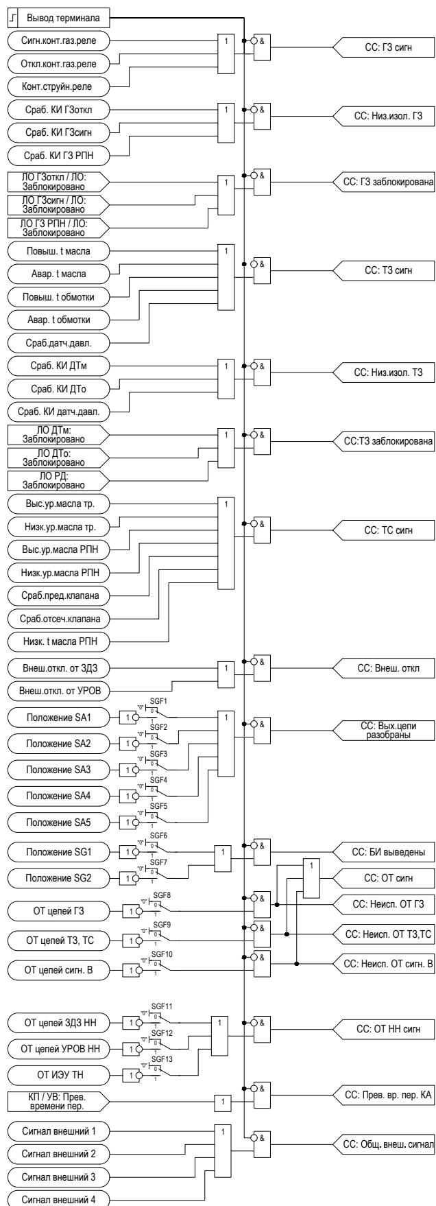
Рисунок 2.36 – Функциональная схема «СС»
