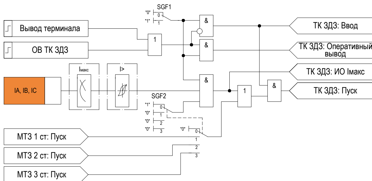
Рисунок 2.9 – Функциональная схема «ТК ЗД3»
